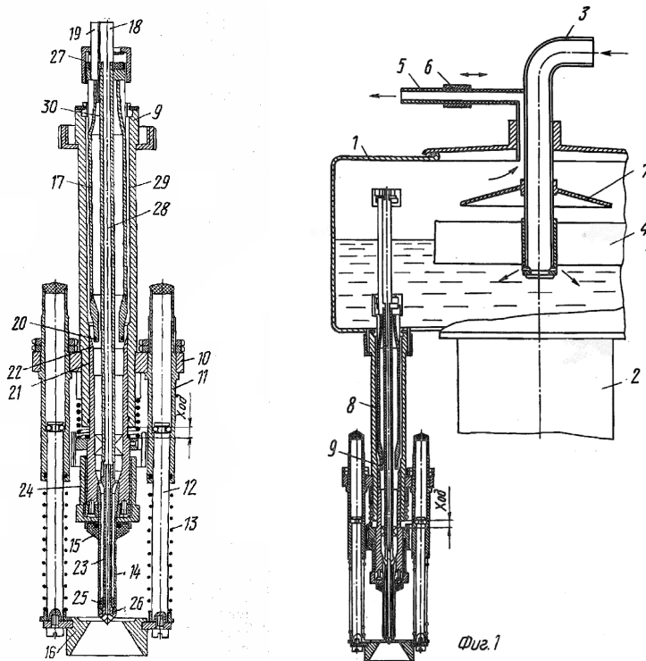
Рис.5 Устройство автоматического дозирования жидких сред.
