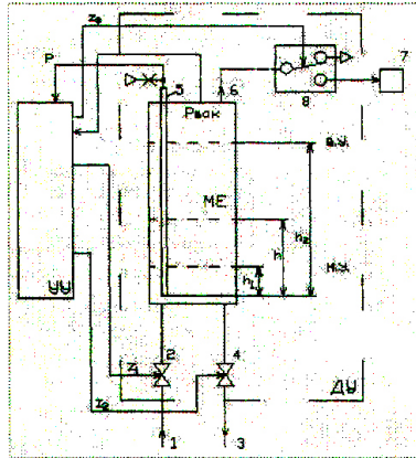
Рис.2 Система весового дозирования
