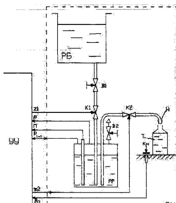
Рис.1 Система объемного дозирования
