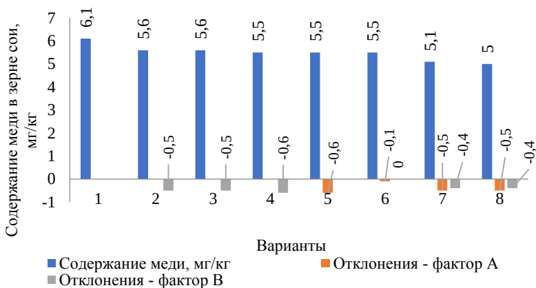
Рисунок 47 – Влияние внесения известкового материала и минеральных удобрений в последствии на содержание меди в зерне сои, 2020 г.
